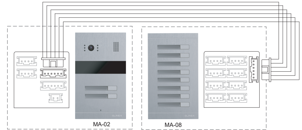
Схема 4. Подключение МА-02 и МА-08.
