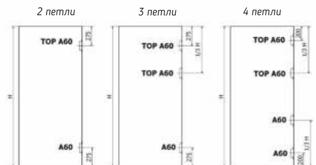
РЕКОМЕНДУЕМОЕ РАСПОЛОЖЕНИЕ ПЕТЕЛЬ В ЗАВИСИМОСТИ ОТ КОЛИЧЕСТВА
